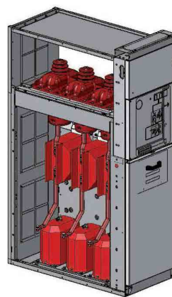
سلول سکسیونر قابل قطع - کوپلینگ SDS-Unit with switch-disconnector - disconnection
