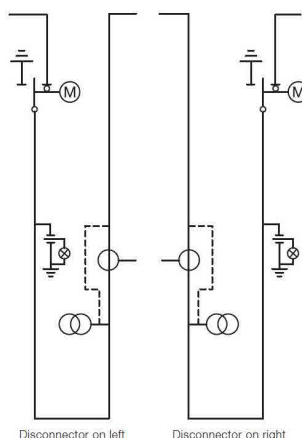
سلول سکسیونر قابل قطع با لوازم اندازه گیری - کوپلینگ SDM - Disconnecting unit with measurements with switch-disconnector
