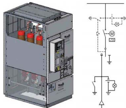
سلول دژنکتوری معکوس SBR – Inverted circuit-breaker unit
