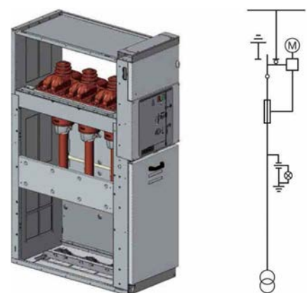
سلول با سکسیونر قابل قطع فیوزدار و لوازم اندازه گیری SFV – Switch-disconnector with fuses – measurements
