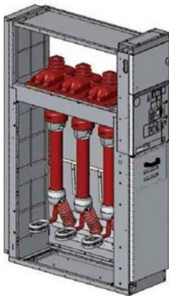
سلول با سکسیونر قابل قطع فیوزدار – کوبلینگ SFS – Switch-disconnector with fuses disconnection –
