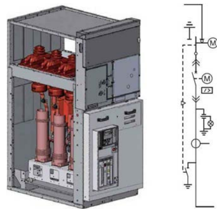
سلول با دژنکتور کشوئی و سکسیونر قابل قطع SBS-W – Withdrawable circuit-breaker unit with switch-disconnector – disconnection
