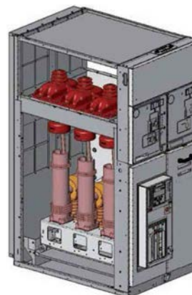
سلول با دژنکتور و سکسیونر قابل قطع – کوبلینگ SBS – Circuit-breaker unit with switch-disconnector – disconnection
