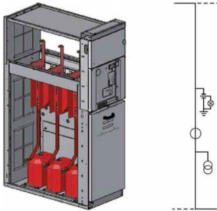
سلول اندازه گیری رایزر DRS – Riser unit - measurements
