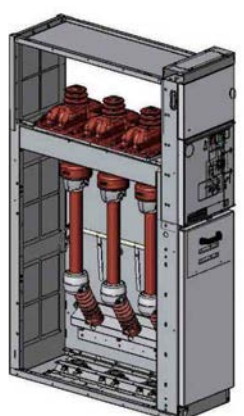
سلول با سکسیونر قابل قطع فیوزدار
